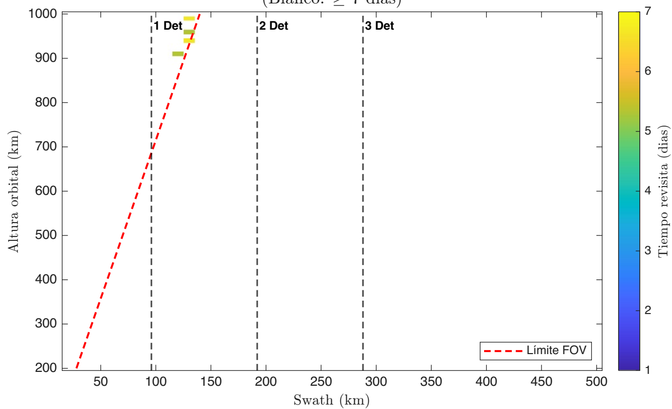
Tiempo Revisita - 3 Satelite(s); 1 Telescopio(s): TMA; Detector 1 (Blanco: \geq 7 dias)
